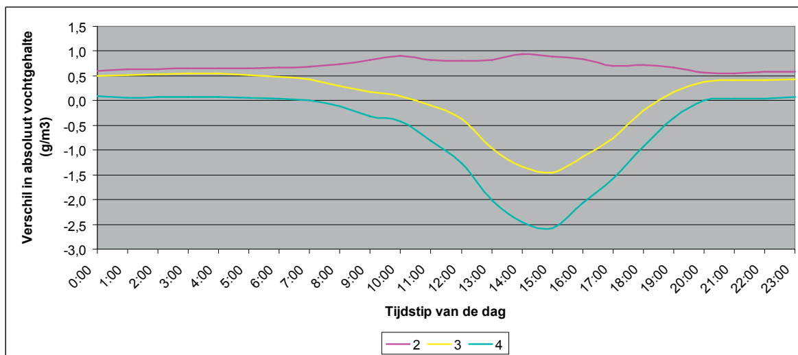
Figuur 28. Cyclisch gemiddelde van 1 april tot 5 juni 2010 van het verschil tussen de absolute luchtvochtigheid onderin en bovenin (g/m 3 ) in drie afdelingen
